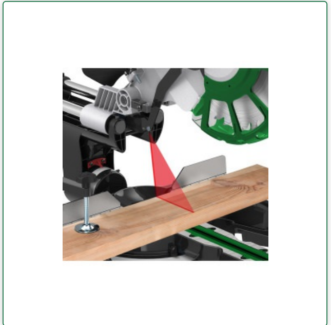
Regulowane szyny oporowe oraz bocznie wysuwane podpory z prawej i lewej strony
